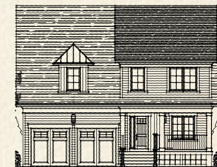
Elevation B
