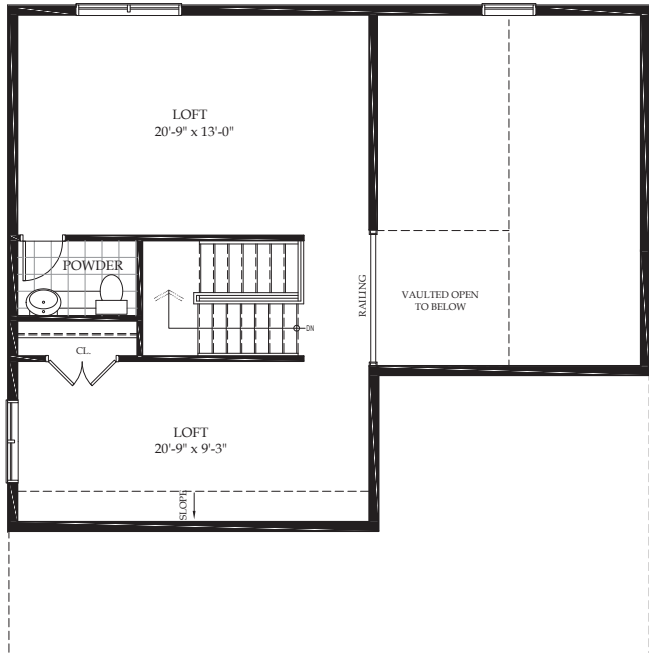
LOFT OPT. A 677 SQ.FT.
